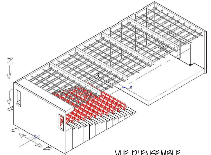
VUE D'ENSEMBLE ISOMETRIQUE
