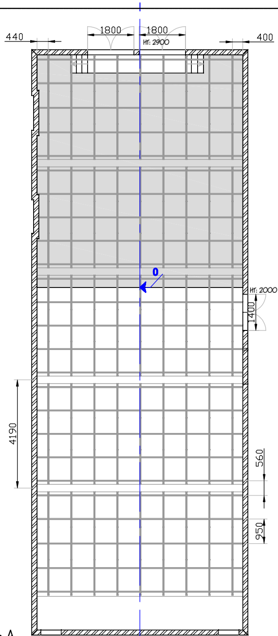
Plan A Vue du grill (tube 50 D)
